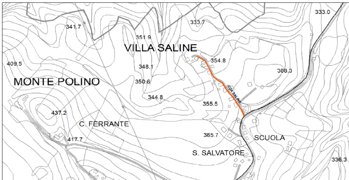
Estratto planimetrico rete gas in Media Pressione da ispezionare nel Comune di Penna San Giovanni: Contrada Saline
