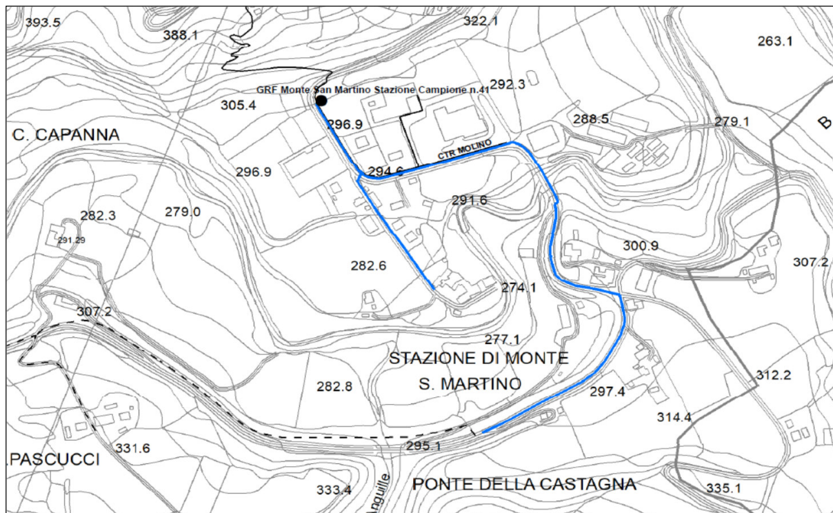
Estratto planimetrico rete gas in Bassa Pressione da ispezionare nel Comune di Monte San Martino: Contrada Molino
